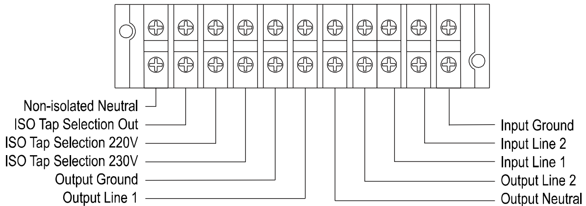
Diagrama de terminales
